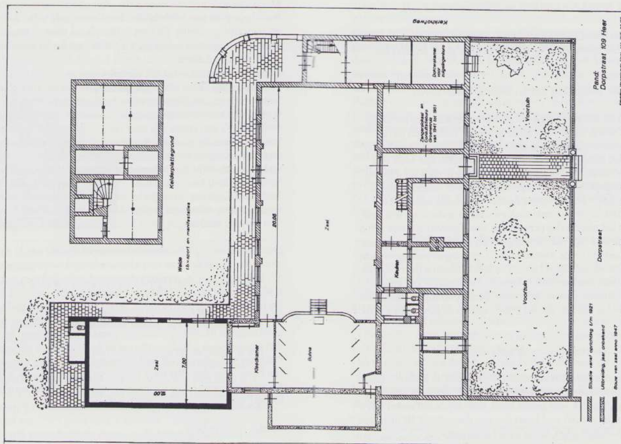
Plattegrond van het voormalige patronaat (en weide), anno 1999
