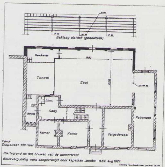
Boven: Reconstructie plattegrond ná verbouwing 1921
